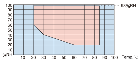
溫度可控制曲線圖例
