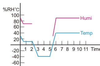
可程式溫溼度圖例
